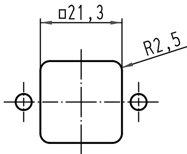
Montageausschnitt panel cut out
